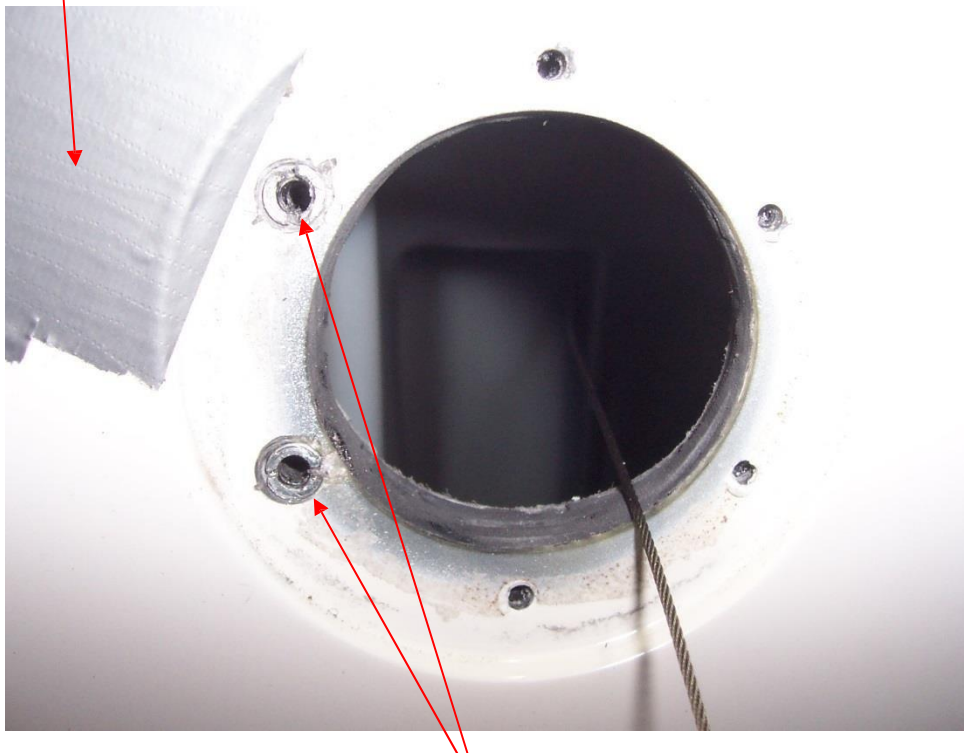
图 6:两个铆接螺帽头，上面有钻孔用固定槽
