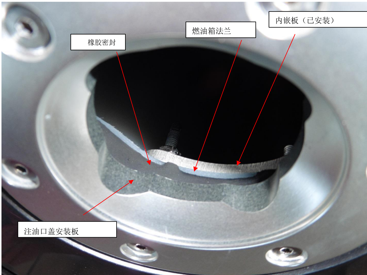
图9: 燃油注油口及其内嵌环与橡胶密封
